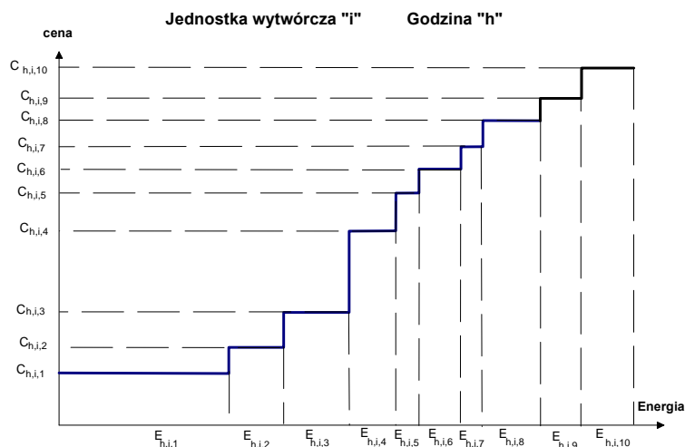
Rys. Z.1. Przykład sposobu przydzielania zmiennych pasmom Oferty Bilansującej
